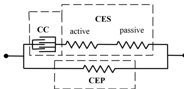
Figure III.2.8. Représentation schématique du modèle de Hill (1938). CC : composante contractile, CES : composante élastique en série, CEP : composante élastique parallèle.
