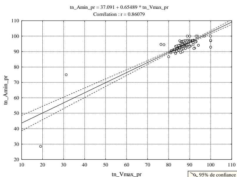
Figure 31 : Relation entre les instants normalisés des pics de vitesse et de freinage du pied arrière
