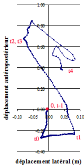
Figure 22 : Déplacement du centre des pressions dans le plan du sol Exemple pour un essai en condition U, réponse à une distance M de l'adversaire.
