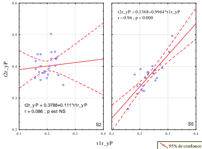
Figure 29 : Relation entre l’instant du poser avant et l’instant du lever arrière
