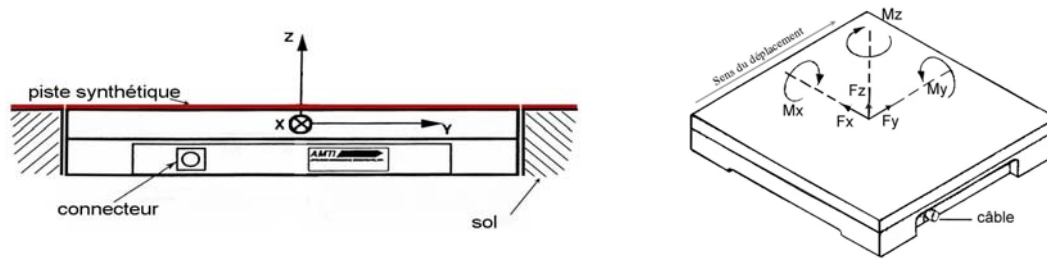
Figure 2. Vue schématique de profil et de \frac{3}{4} dessus de la plateforme de force AMTI intégrée au sol
