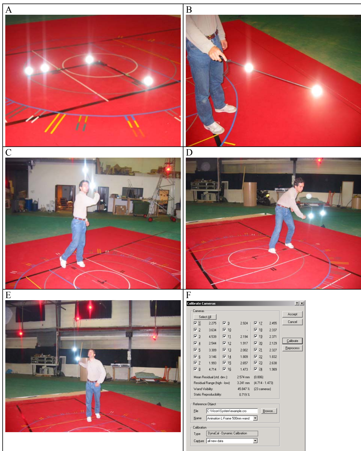
Figure 6 : Equerre utilisée pour la calibration statique (A). Baguette utilisée pour la calibration dynamique (B). Mouvements de la baguette permettant au système de reconstruire la métrique du volume de travail (C-E). Résultats de la calibration (F).
