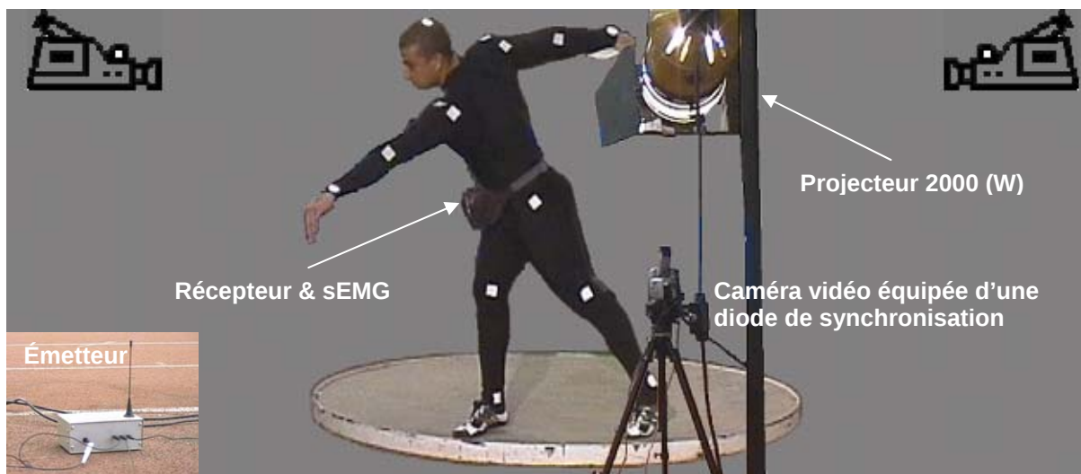
Photo 4-3 : Lanceur équipé
