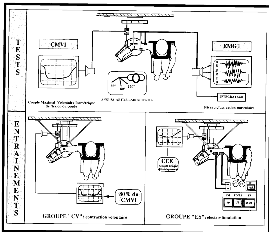
Figure 2 - Dispositif ergométrique.
